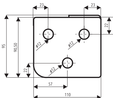
Pohled zepředu
